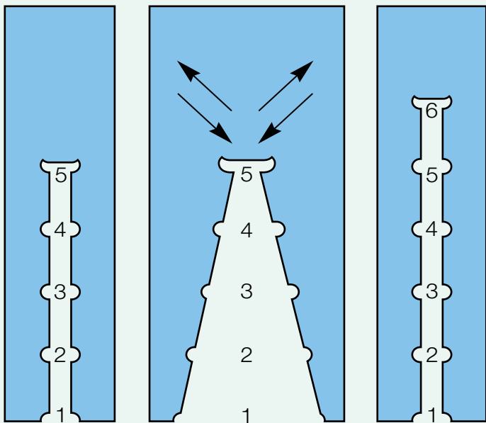
Rissentstehung je Biegezyklus
