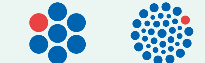
Vergleich der Querschnittsfläche eines Drahtes in einer 7-drähtigen Litze zu einer Warrington-Seale Litze mit 36 Drähten
