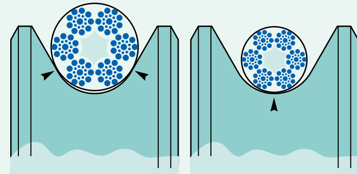
Pressung an den Flanken bei zu kleiner Rille – das Seil wird drehen
