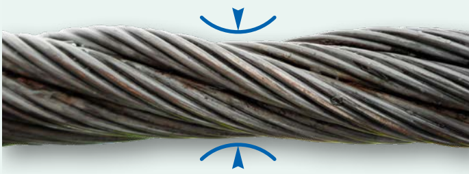
Eingefallener Stoss im Spleiss
