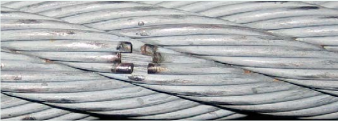
Häufung von Drahtbrüchen – kann sehr gut magnetinduktiv erkannt werden
