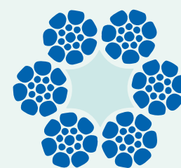
Verdichtetes Seil 6×15 Seale
