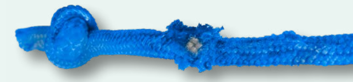
Klassische Scheuerstelle eines Bügelseils am Austritt oberhalb des Knotens
