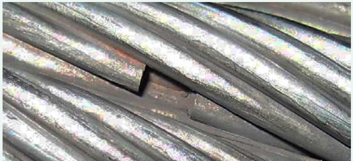
Klassisches Erscheinungsbild im Seilbahnseil
